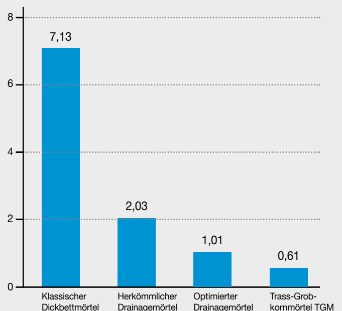
Vergleich Wasseraufnahme verschiedener Verlegemörtel in %
